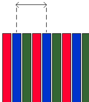
DENSIDAD DE REJILLA DE APERTURA EN UNA UNA MASCARA DE RANURA
