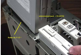
Fig. 13-1 Rail de CD-ROM
