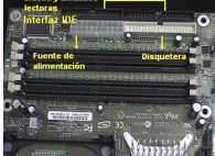
Fig 8 Conectores internos
